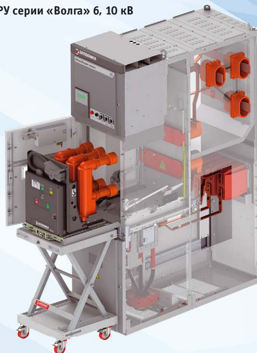
Малогабаритное КРУ серии «Волга» 6, 10 кВ
