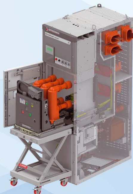
Малогабаритное КРУ серии «Волга» 6, 10 кВ
